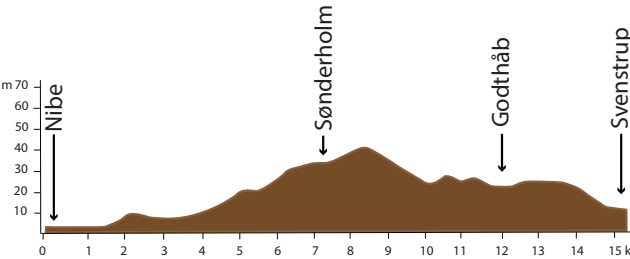
Længdesnit over strækningen fra Nibe til Svenstrup
